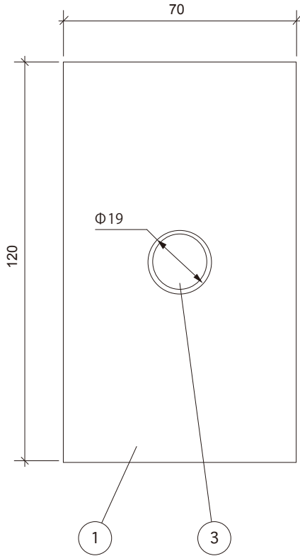
■ 正面図
