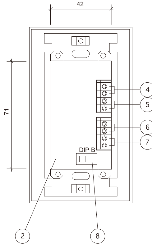
■ 背面図
